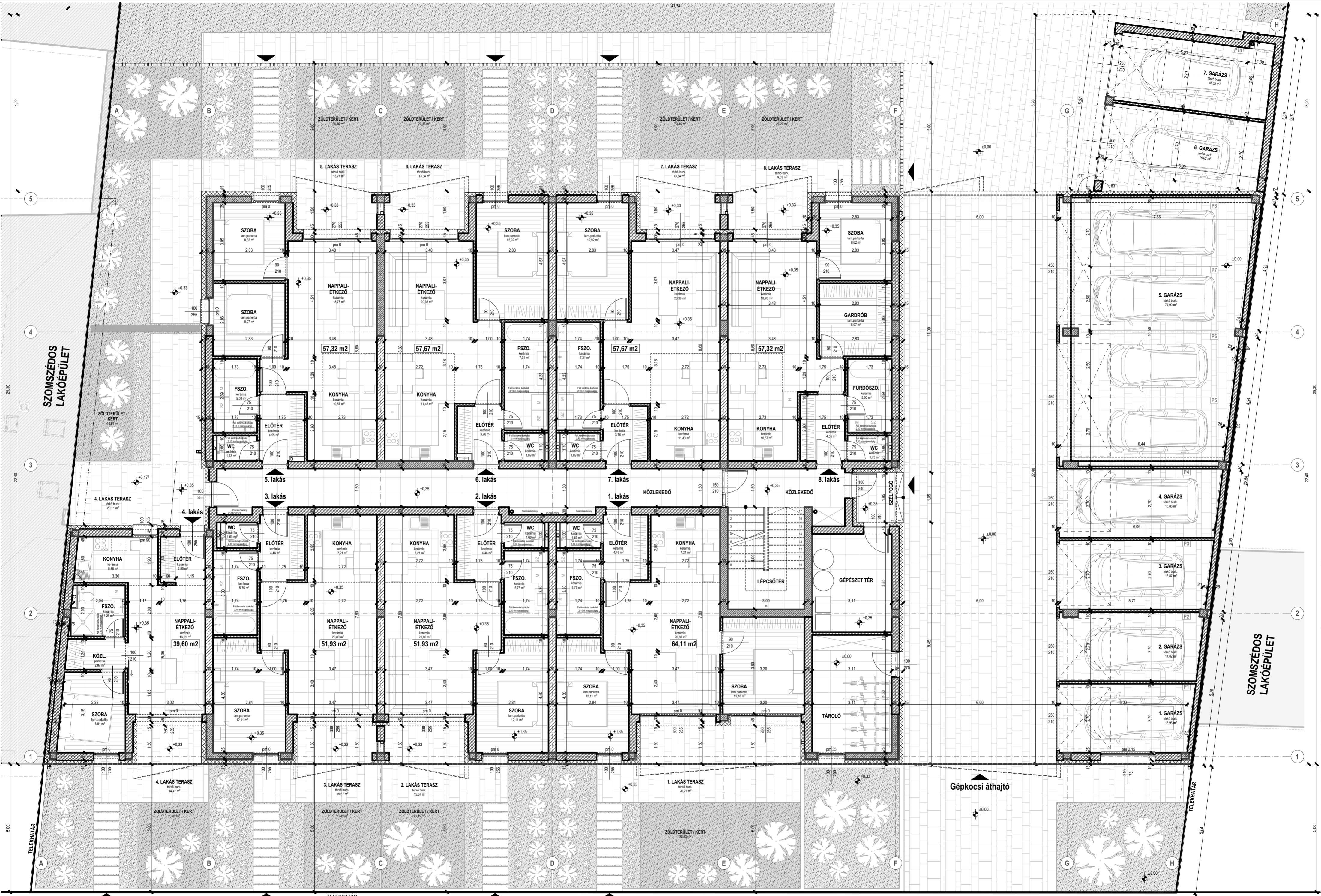
HAJDÚSZOBOSZLÓ, SZURMAI UTCA 4-6. SZ. - FÖLDSZINTI ALAPRAJZ
